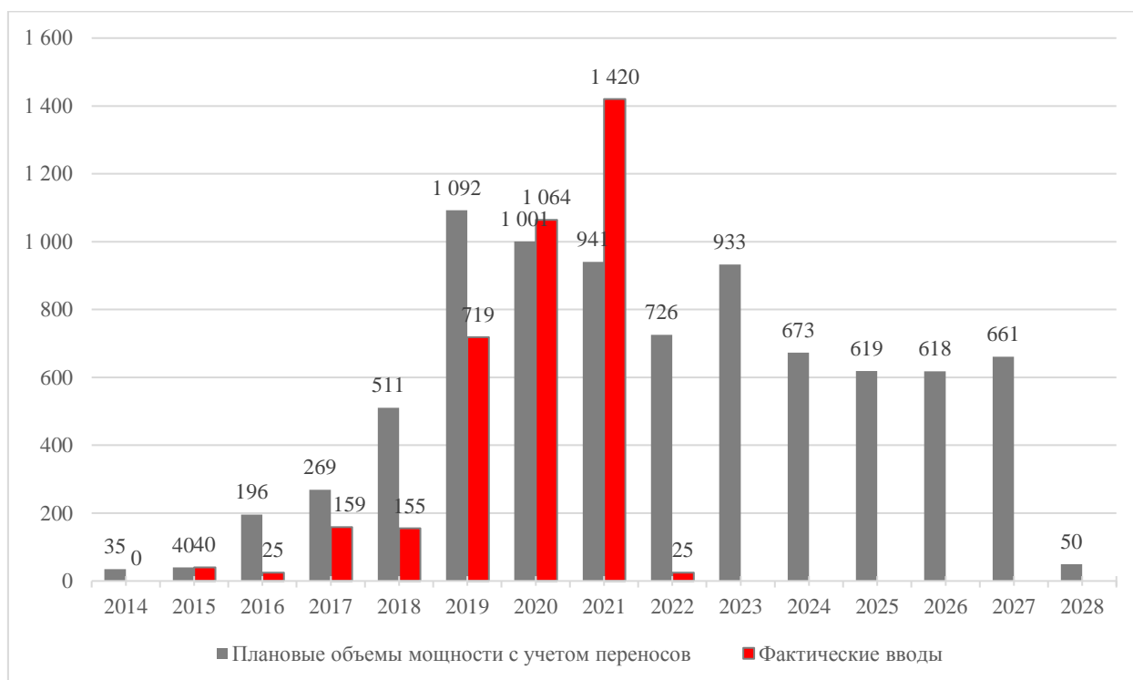
Рис. 2 «Плановые и фактические показатели ввода мощности в 2014-2028 гг. с учетом ввода объектов генерации, запланированных к вводу в предыдущие годы, МВт» 1 .
