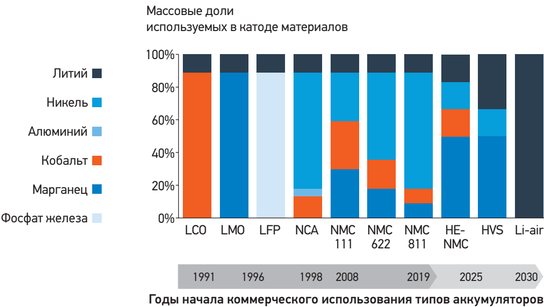
Рис. 14. Технологическое развитие литий-ионных аккумуляторов (год начала коммерческого использования)
